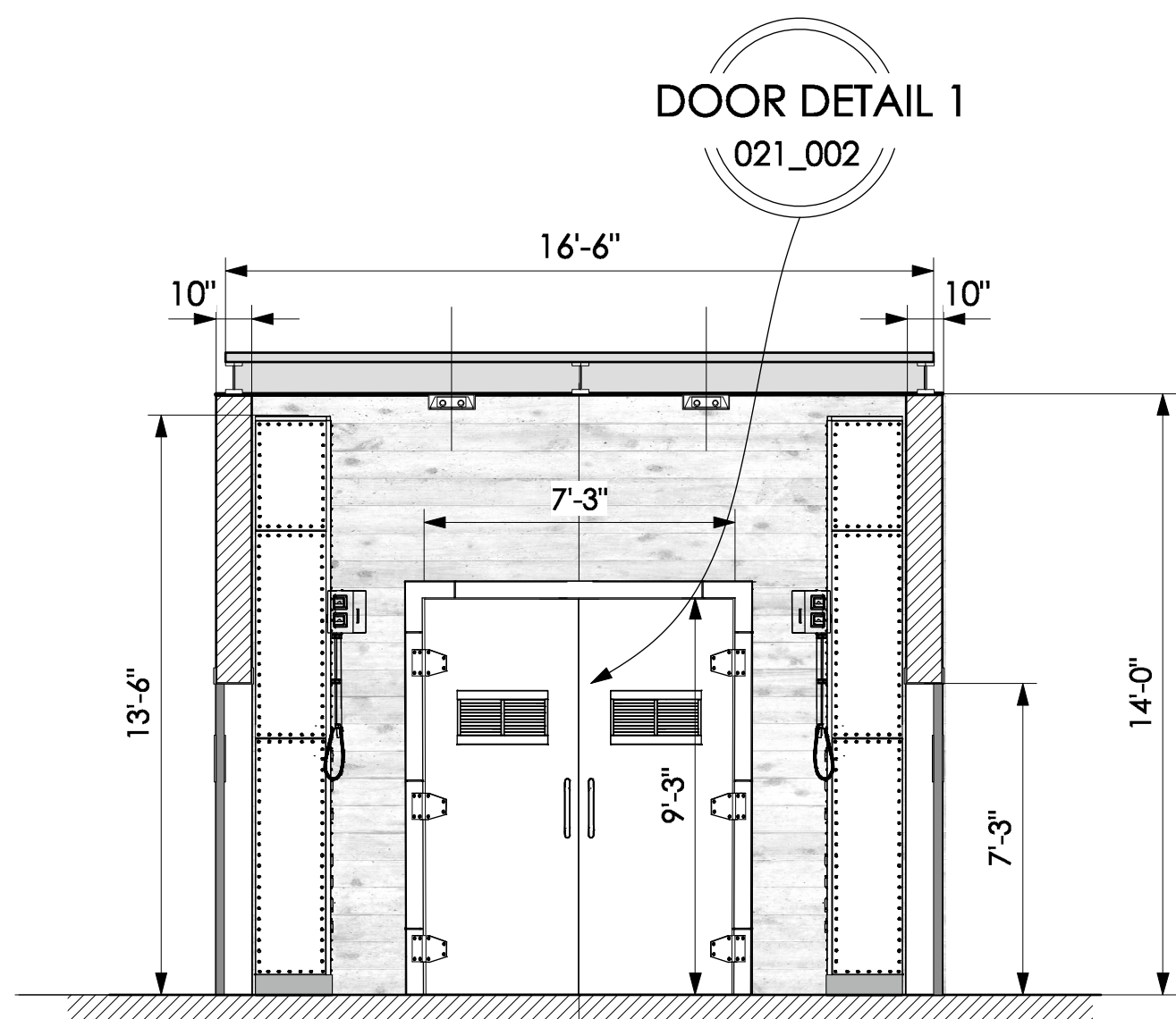
ELEVATION B-B
