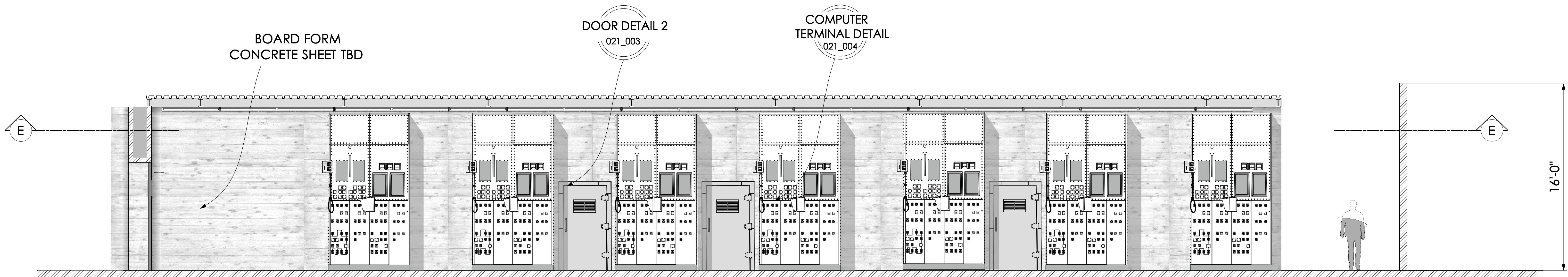
ELEVATION A-A
