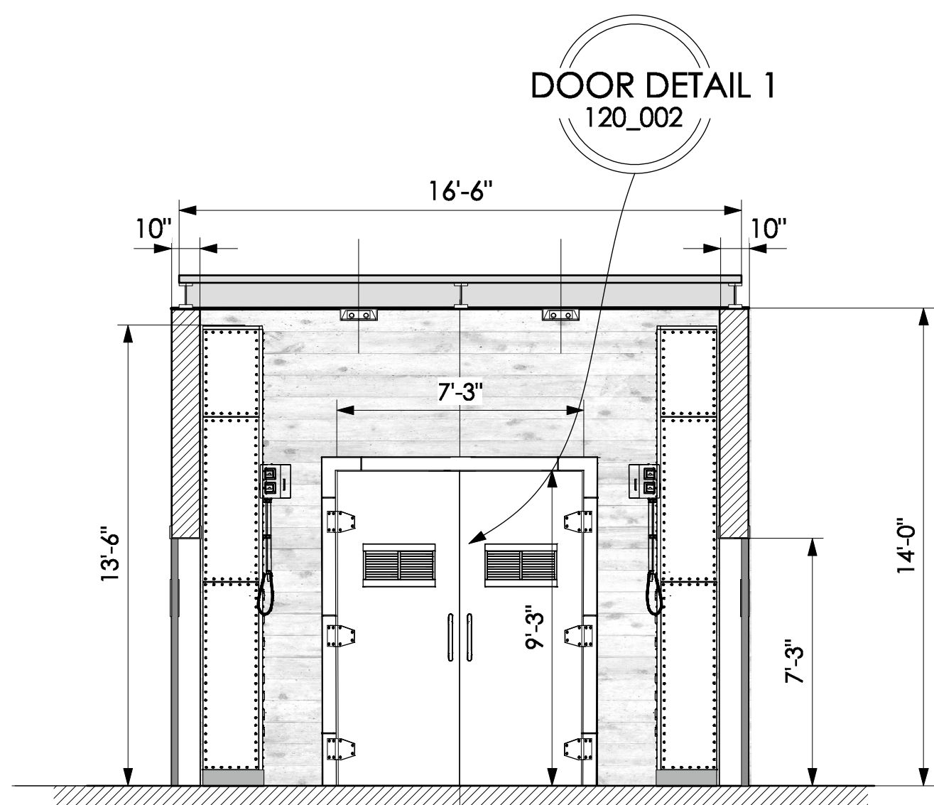
ELEVATION B-B
